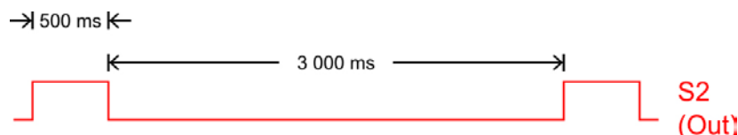
Abbildung 22: Zyklischer Überstromimpuls.
