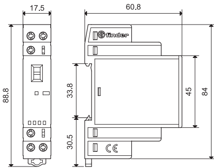
Typ 22.34 Schraubklemmen
