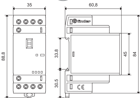
Typ 22.44 / 22.64 Schraubklemmen
