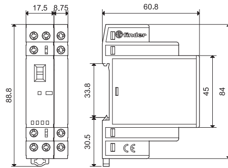
Typ 22.34 + 022.33 / 022.35 Schraubklemmen
