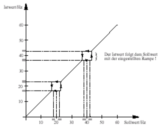
Bild 9.5.1 Drehfeldfrequenz bei Verwendung der Ausblendfrequenz
