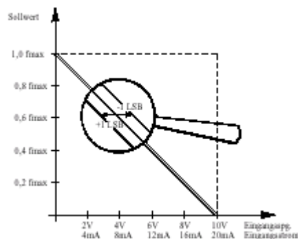
Bild 9.3.2 Sollwert- Offset bei 10-0V, 20-0mA Sollwertvorgabe
