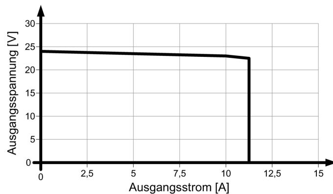
Bild 6-6 Ausgangskennlinie 6EP3334-8SB00-0AY0 Parallelbetrieb
