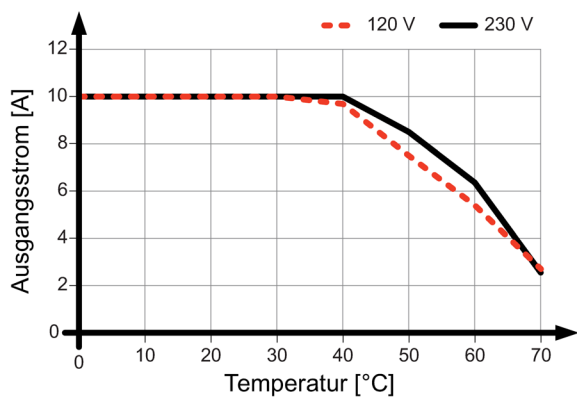
Bild 4-13 6EP3334-8SB00-0AY0 Einbaulage (5)
