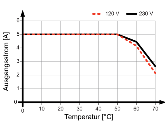
Bild 4-8 6EP3333-8SB00-0AY0 Einbaulage (5)
