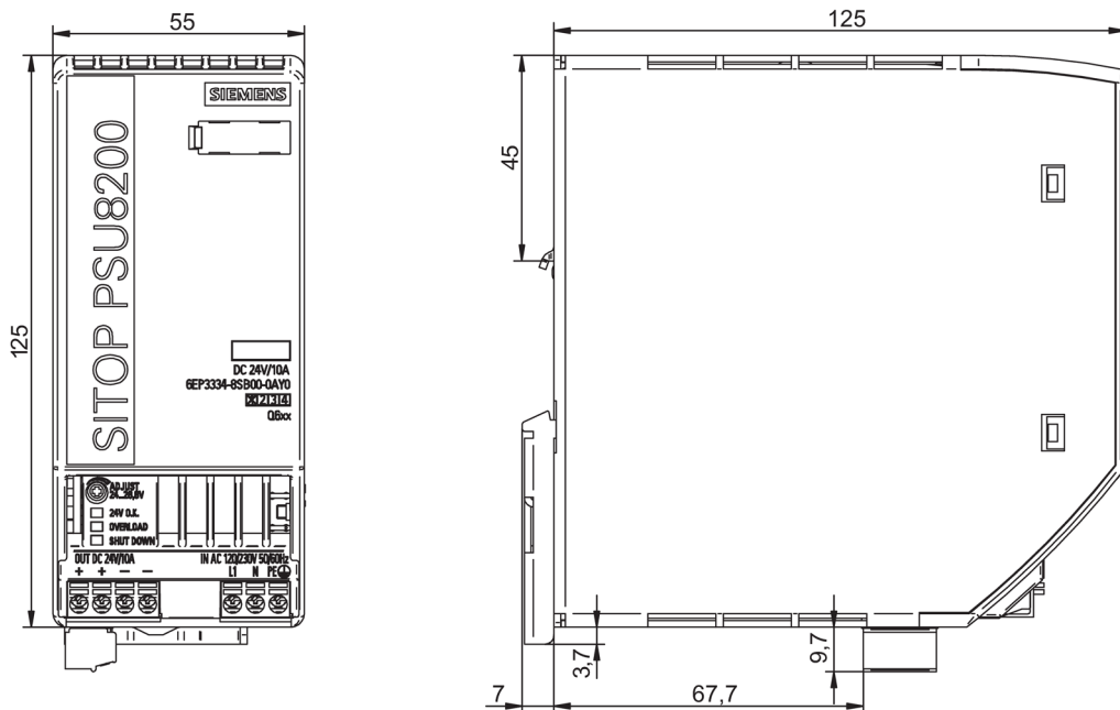
Bild 2-9 Maßzeichnung 6EP3334-8SB00-0AY0
