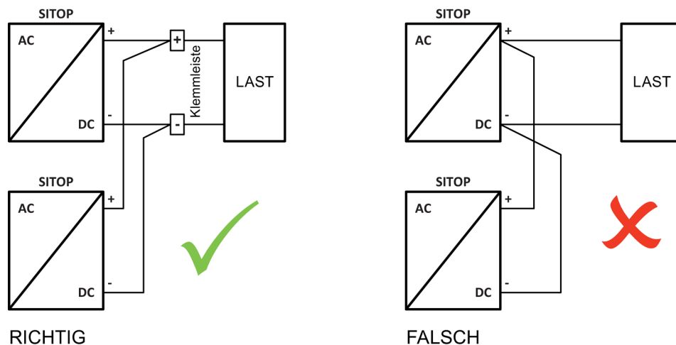
Bild 9-1 Parallelschaltung
