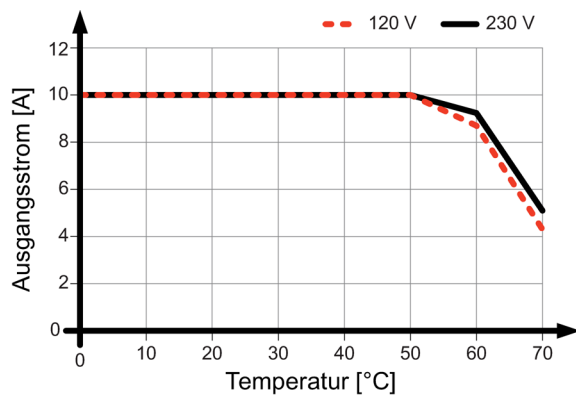
Bild 4-11 6EP3334-8SB00-0AY0 Einbaulage (3)
