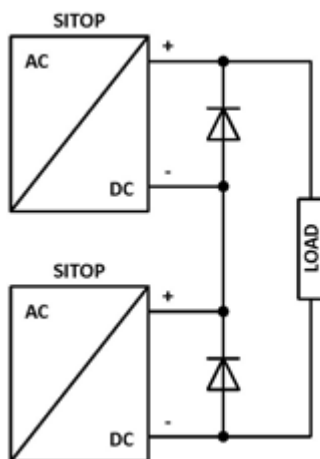
Bild 9-3 Reihenschaltung
