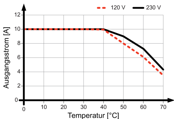
Bild 4-12 6EP3334-8SB00-0AY0 Einbaulage (4)
