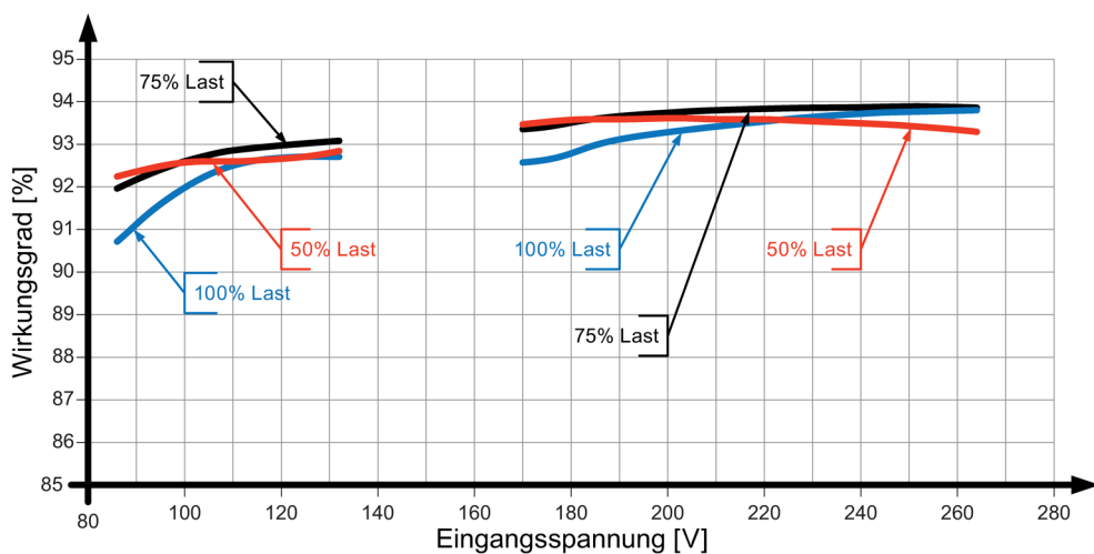
Bild 6-10 Wirkungsgrad 6EP3334-8SB00-0AY0
