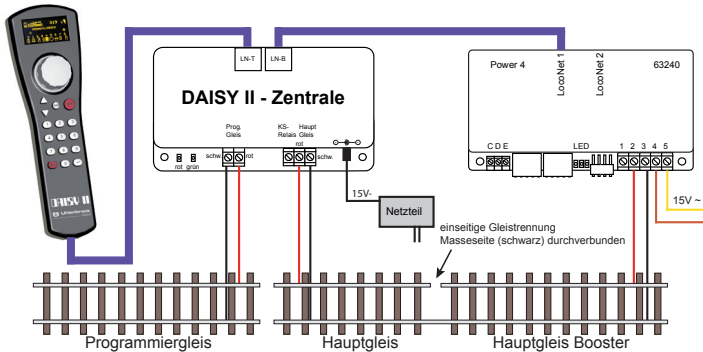
Anschlusssskizze eines Boosters
