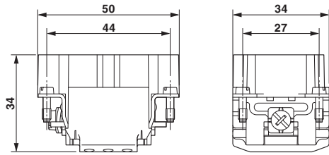
Maßzeichnung
