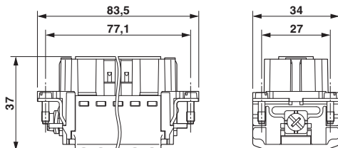
Maßzeichnung
