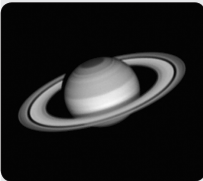
Abb. 44a: Der Planet Saturn, hier nun mit einer höheren Vergrößerung abgebildet. Deutlich sind die Ringteilungen zu erkennen. Saturn hat die größten Ringe im Sonnensystem.
