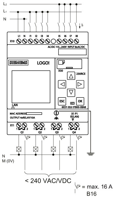
Zweiphasiger Anschluss des Basismoduls
