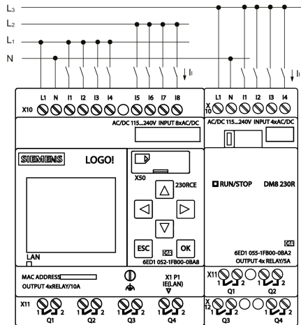
Dreiphasiger Anschluss des Basismoduls an ein Erweiterungsmodul
