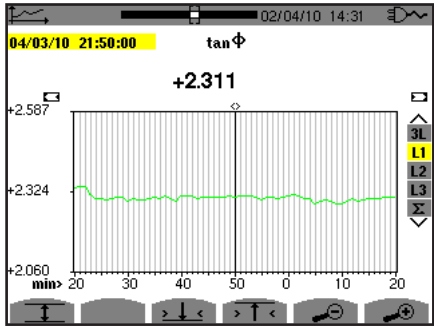
Abbildung 85: tan \Phi (L1) ohne MIN-AVG-MAX für eine dreiphasige Quelle mit Neutralleiter
