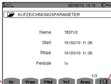
Abbildung 78: Bildschirm Aufzeichnungs-Eigenschaften
