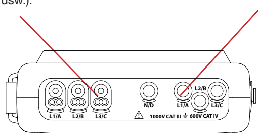
Abbildung 4: Anschlussbuchsen
