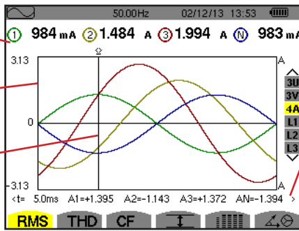
Abbildung 55: Bildschirm zur RMS-Anzeige bei 4A
