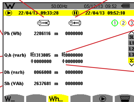
Abbildung 104: Bildschirm zur Anzeige der verbrauchten und erzeugten Energien Gesamtenergien bei \Sigma
