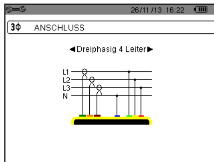
Abbildung 25: Menü Anschluss
