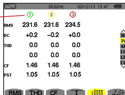
Abbildung 68: Bildschirm zur gleichzeitigen Anzeige bei 3V
