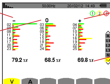
Abbildung 50: Bildschirm des Expertenmodus für die Phasenspannung (dreiphasige Anordnungen mit Neutralleiter)
