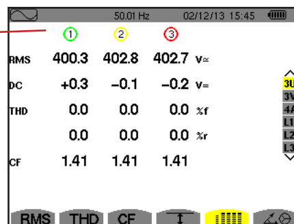
Abbildung 67: Bildschirm zur gleichzeitigen Anzeige bei 3U
