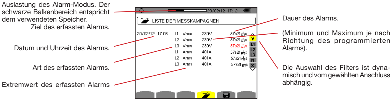
Abbildung 75: Bildschirm Alarm-Liste
