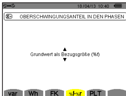
Abbildung 24: Menü Wahl der Oberschwingungsgehalt-Bezüge
