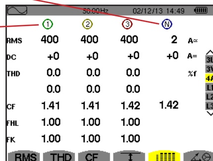
Abbildung 69: Bildschirm zur gleichzeitigen Anzeige bei 4A
