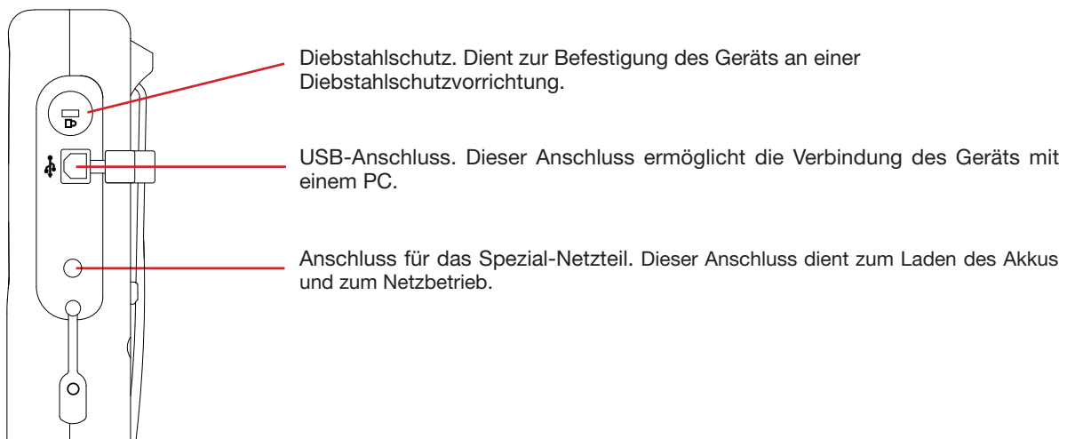
Abbildung 5: Seitliche Anschlüsse
