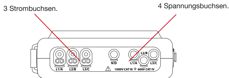
Abbildung 11: Anschlussbuchsen
