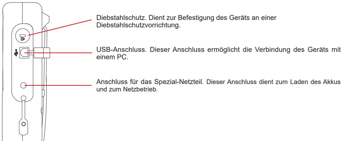
Abbildung 4: Seitliche Anschlüsse
