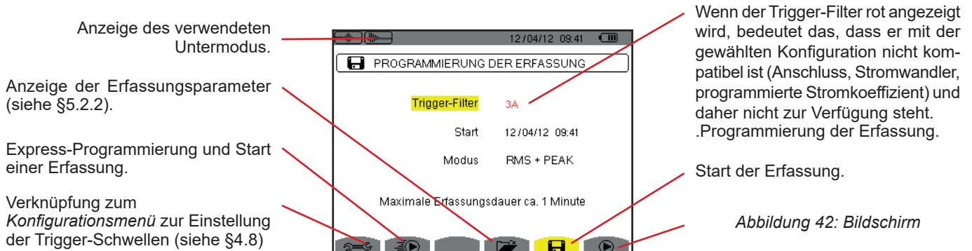
Programmierung der Erfassung im Modus Anlaufstrom
