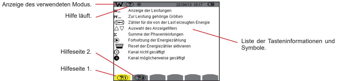
Abbildung 121: Beispiel der Hilfeseite für den Modus Leistungen und Energien, Seite 1
