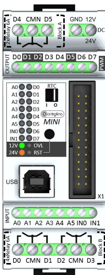
Abbildung 1: CONTROLLINO MINI
