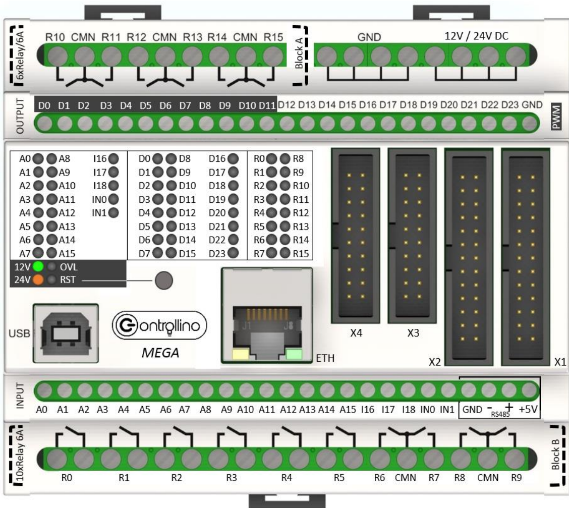
Abbildung 3: CONTROLLINO MEGA
