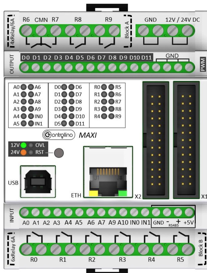
Abbildung 2: CONTROLLINO MAXI
