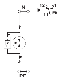
Schaltplan
