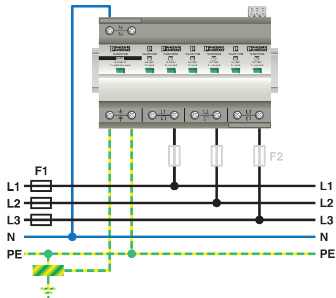
Applikationszeichnung
