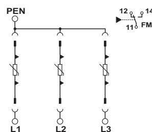
Schaltplan
