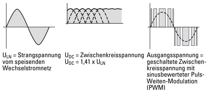
Blockschaltbild mit Hauptkomponenten eines Frequenzumrichters
