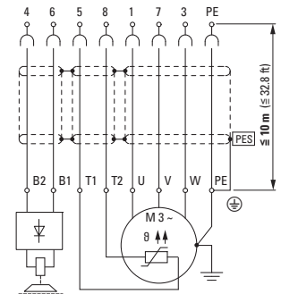
Beispiel: Motorabgang mit geschirmter Motorleitung bei RASP
