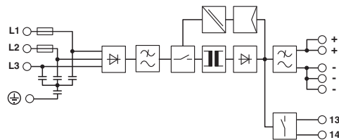
Blockschaltbild
