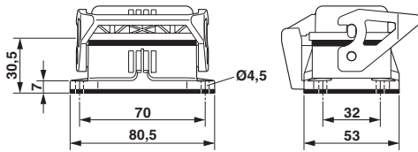
Maßzeichnung
