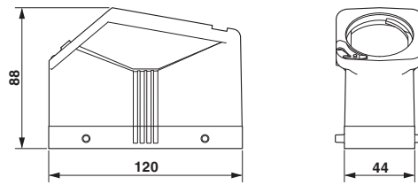
Maßzeichnung
