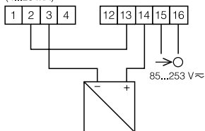
Abb. 5. Anschlussweise des Messgeräts.
