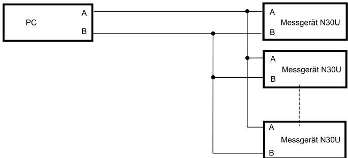
Abb. 12. Anschlussweise der RS-485-Schnittstelle.
