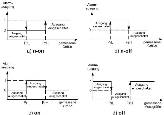
Abb. 11. Alarmtypen: a) n-on, b) n-off c) on d) off.
