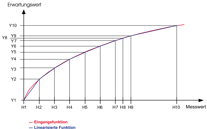
Abb. 10. Individuelle Kennlinie.
