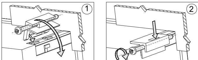
Abb. 2. Befestigung des Messgeräts
