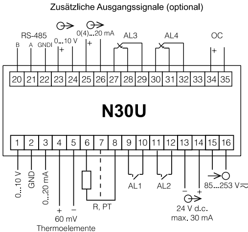
Abb. 4. Beschreibung der Signale auf den Anschlussleisten.
