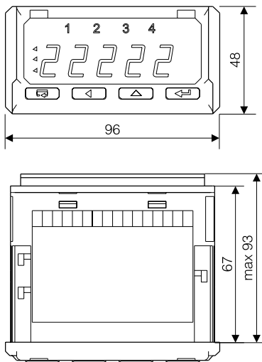
Abb. 3. Maßbild des Messgeräts
