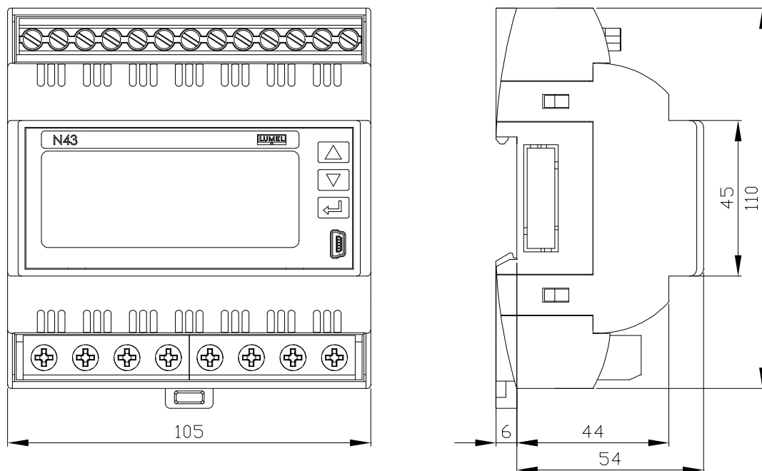
Abb. 1. Abmessungen des Messgerätes
