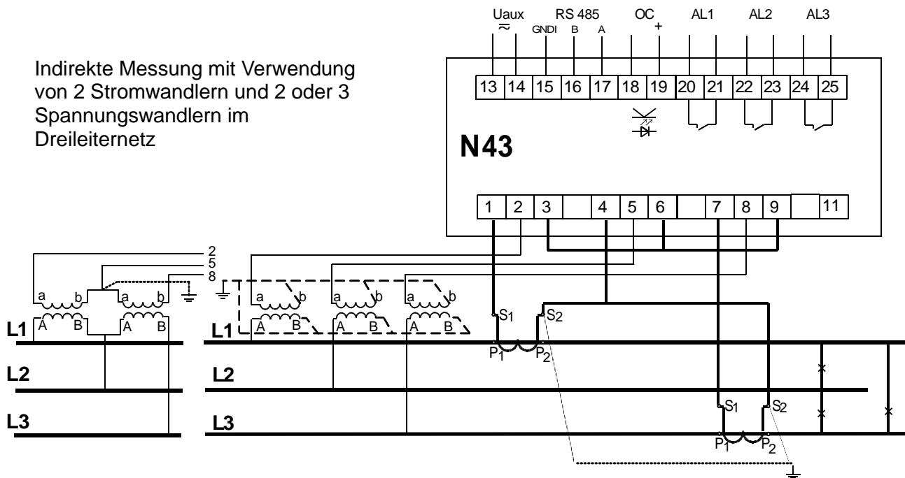
Abb. 2. Anschlusspläne des Messgerätes im Netz: a) Dreiphasenstrom-Vierleiternetz, b) Dreiphasenstrom-Dreileiternetz
