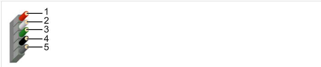
Fig. 5 Standard Kabelbelegung 1x5 Buchsenleiste
