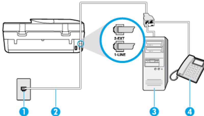
Abbildung B-18 Rückansicht des Druckers
