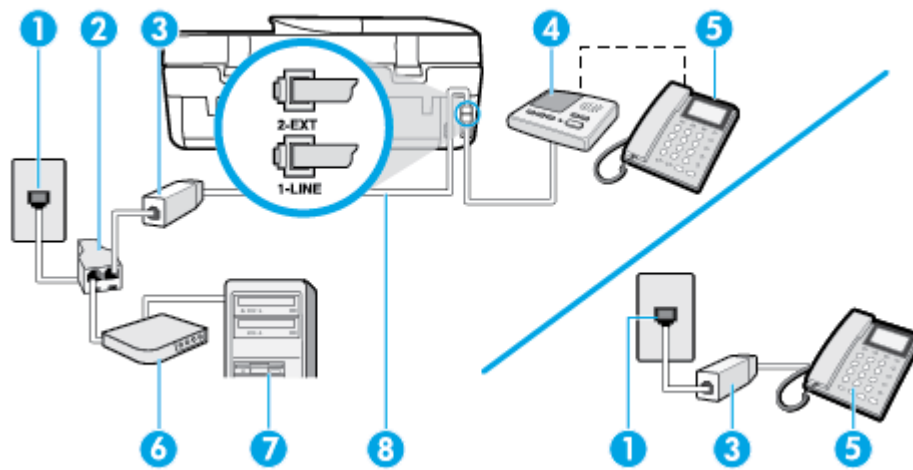
Abbildung B-15 Rückansicht des Druckers
