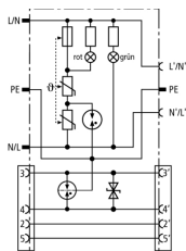
Principalschaltbild DPRO 230 NT
