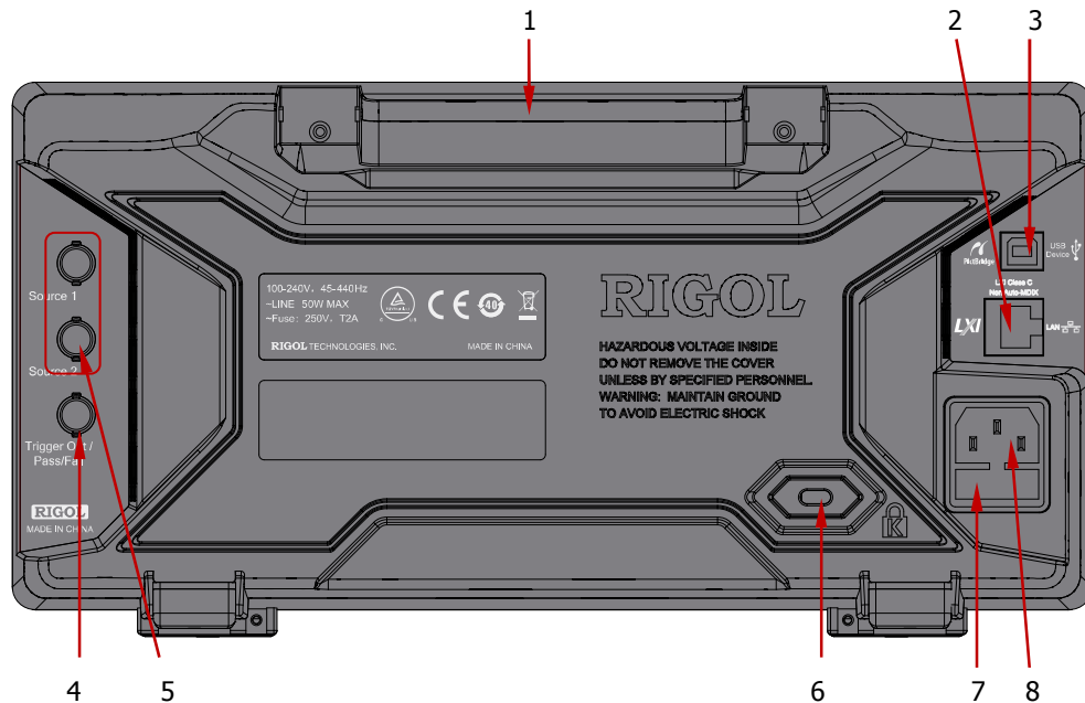
Bild 1-10 Rückseite Übersicht
