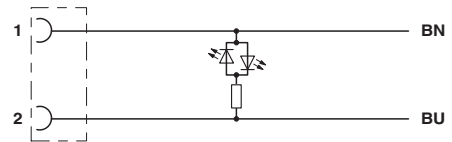
Kontaktbelegung des DEUTSCH DT06-2S
