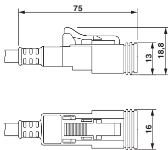
Maßzeichnung
