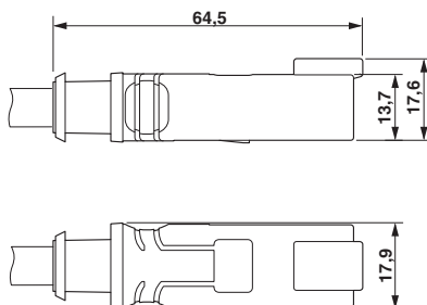
DEUTSCH DT04-2P, Drauf- und Seitenansicht
