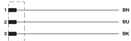
Kontaktbelegung des DEUTSCH DT04-3P
