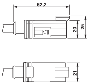
Maßzeichnung
