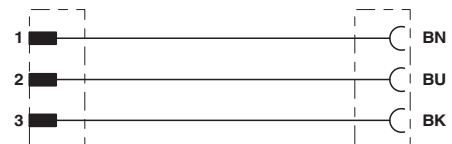
Kontaktbelegung der DEUTSCH-Steckverbinder
