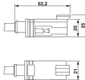
DEUTSCH DT04-3P, Drauf- und Seitenansicht
