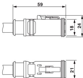
DEUTSCH DT06-3S, Drauf- und Seitenansicht
