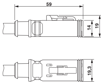
Maßzeichnung
