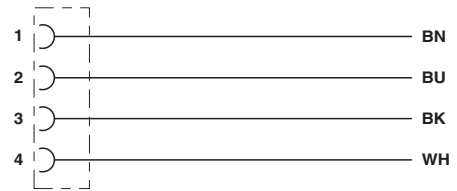
Kontaktbelegung des DEUTSCH DT06-4S
