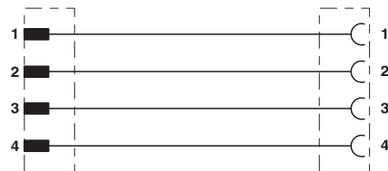
Kontaktbelegung der DEUTSCH-Steckverbinder
