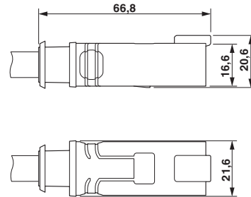
DEUTSCH DT04-4P, Drauf- und Seitenansicht
