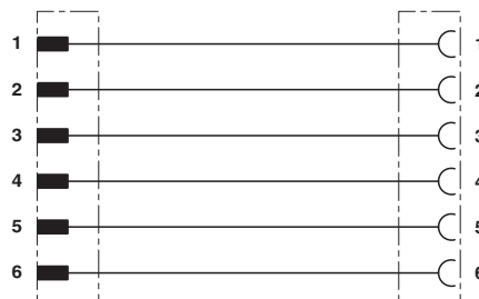
Kontaktbelegung der DEUTSCH-Steckverbinder
