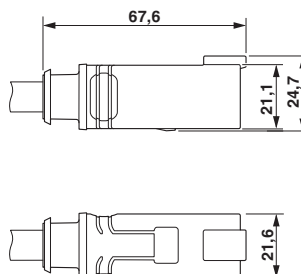
DEUTSCH DT04-6P, Drauf- und Seitenansicht
