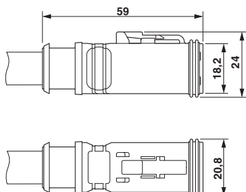
DEUTSCH DT06-6S, Drauf- und Seitenansicht
