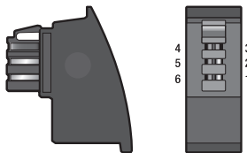
TAE/RJ45-Adapter: Pins des TAE-Steckers
