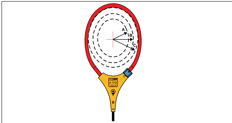
Abbildung 1: Positionsempfindlichkeit
