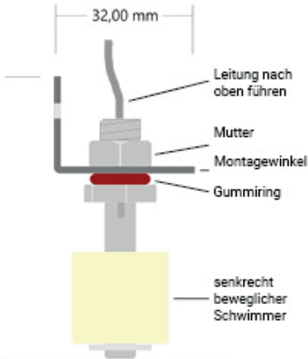
Maßstabsgetreue Zeichnung, am Beispiel mit 200940
