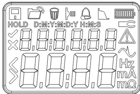
Abbildung 4: DET14C/DET24C Anzeigenseite
