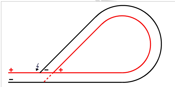
Abb. 1: Kurzschluss-Problematik an der Weiche einer Kehrschleife
