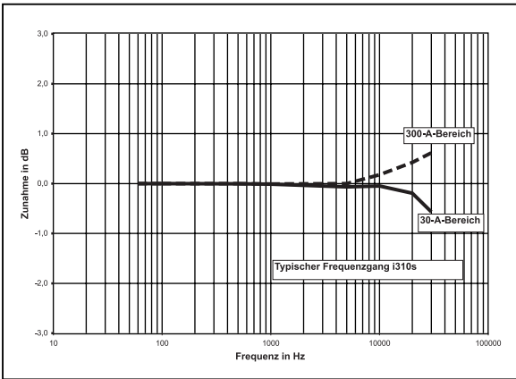
Typischer Frequenzgang
