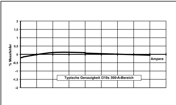
Typische Genauigkeit
