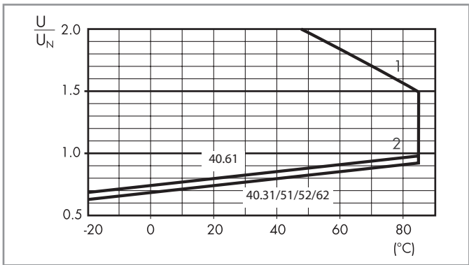
R 40 - DC Spulen-Betriebsspannungsbereich Sensitive Spule, Typ 40.31/51/52/61/62
