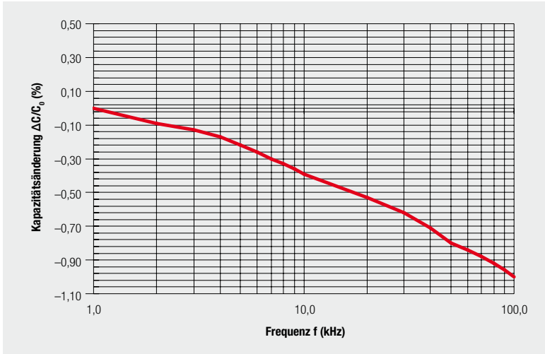
Abb. 2.2: Frequenzabhängige Kapazitätsänderung, Beispiel: MKP Filmkondensator
