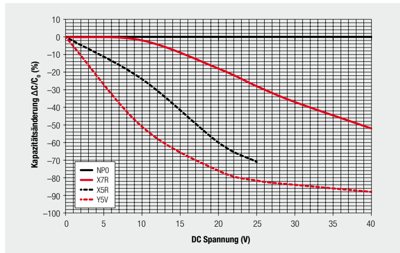
Abb. 2.1: Spannungsabhängige Kapazitätsänderung, Beispiel: Keramik Kondensatoren
