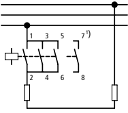
Einphasenleistung AC-1
