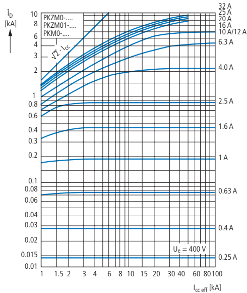
Durchlasswerte Motorschutzschalter
