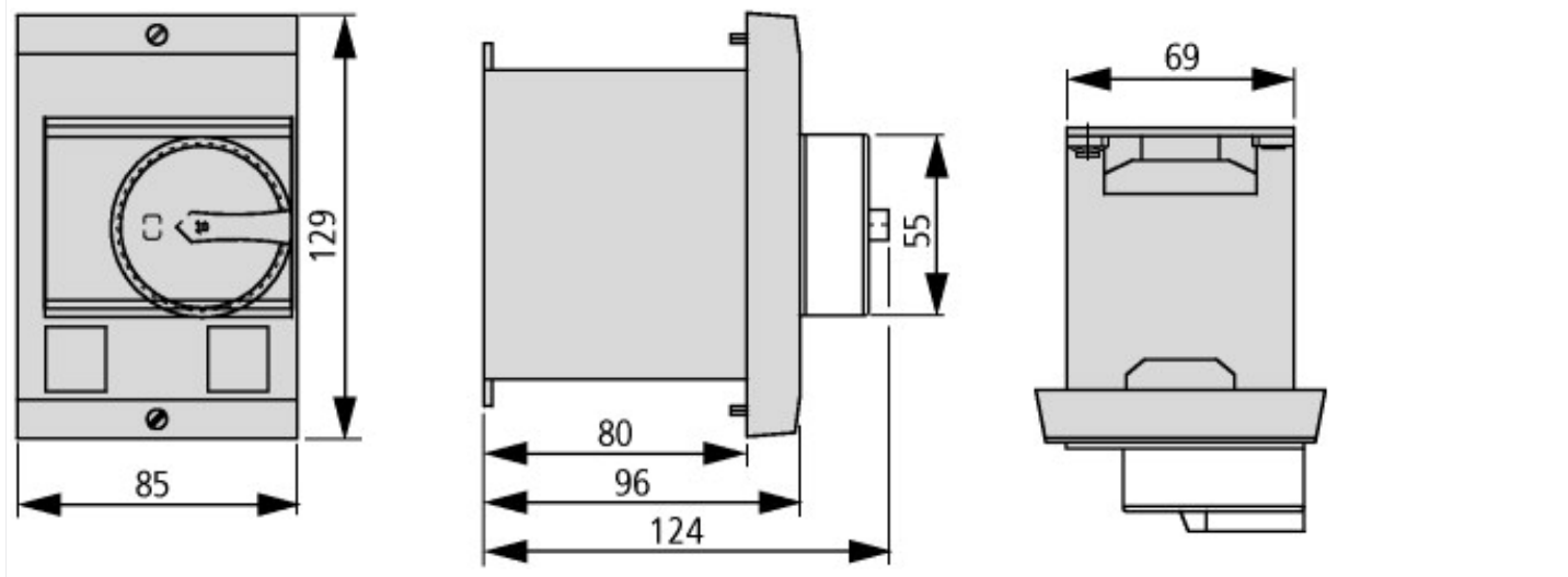
Einbauöffnung E-PKZ0...
