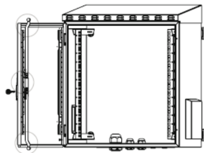
3-Punkt-Verriegelungssystem
