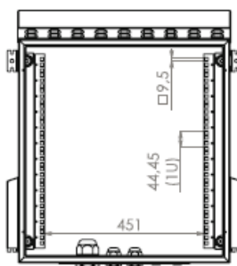
Innenansicht
