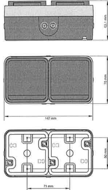
Bild 3: Steckdose SCHUKO 2fach mit Klappdeckel Steckdose
