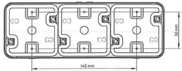
Bild 4: SCHUKO 3fach mit Klappdeckel
