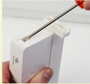
Abb. 21/22: Schutzabdeckung 'RS' ausbrechen
