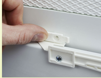
Abb. 4: Fensterrahmen-Halterung (D) mittels Segel anlegen
