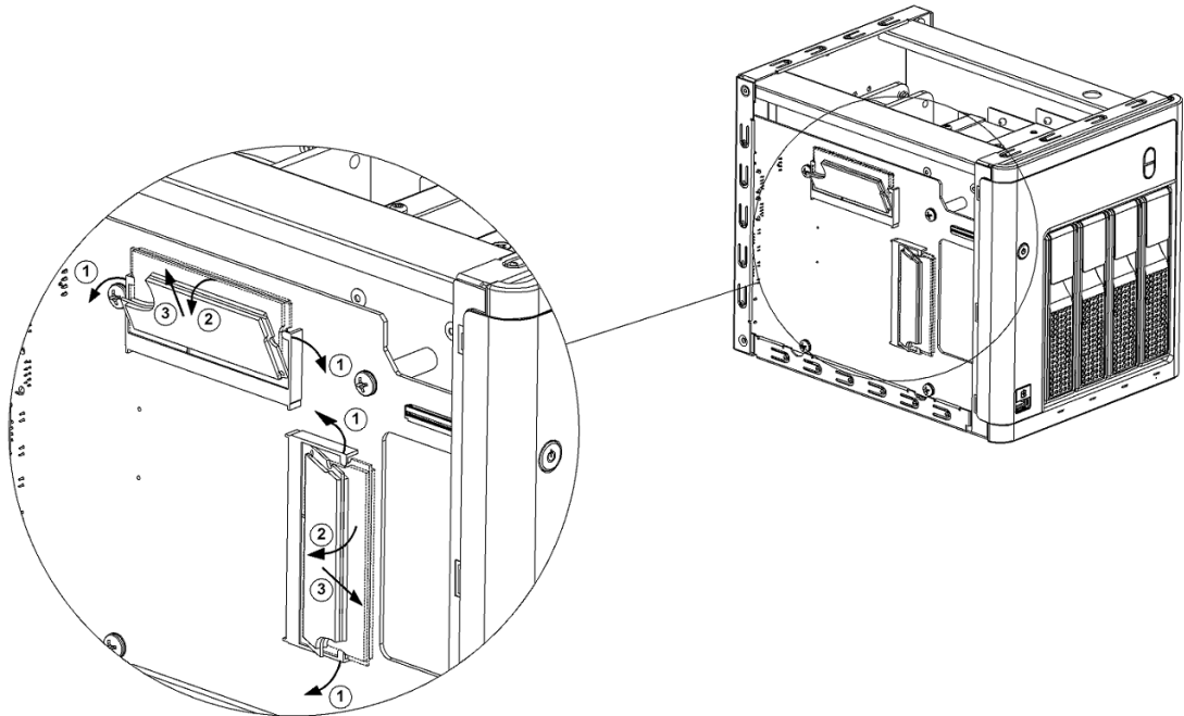
Abbildung 2. 4PL-SODIMM-Modul austauschen
