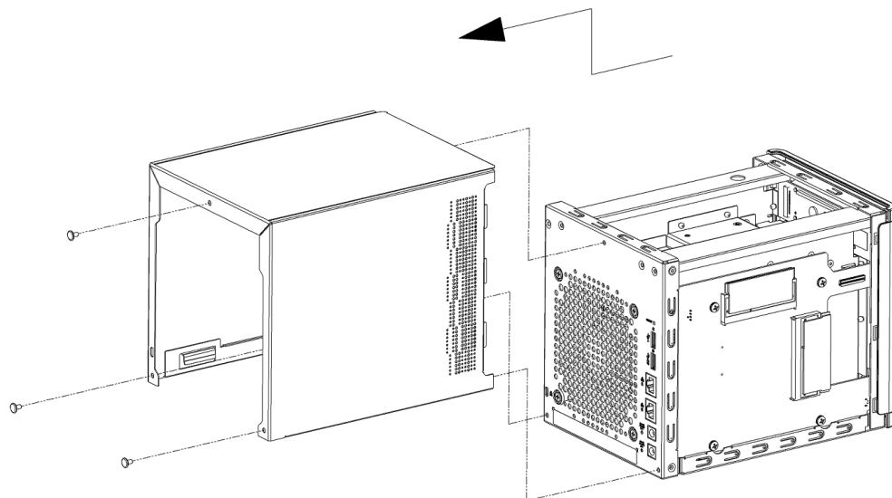
Abbildung 1. Gehäusedeckel der Einheit abschrauben und entfernen
