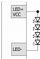
serieller Anschluss von LEDs
