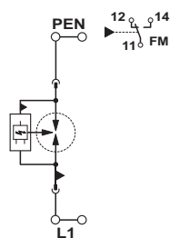
Schaltplan
